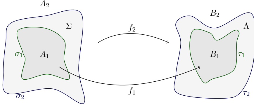
FIGURE 3.1. Cadre de la technique de la modification locale
