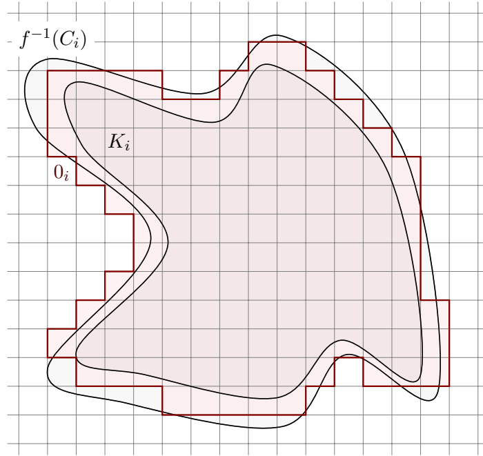
FIGURE 5.1. Construction de l'ensemble O_i
