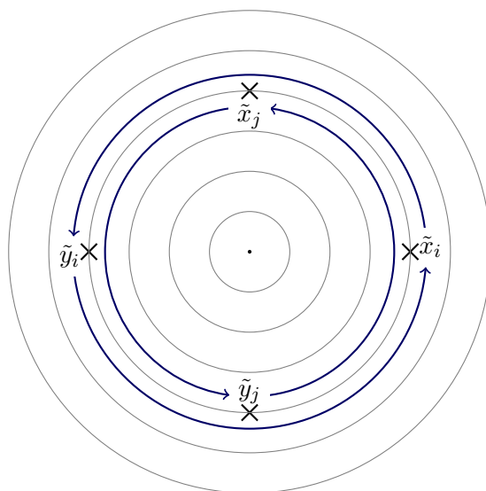
FIGURE 2.2. Homéomorphisme conservatif envoyant \tilde{x}_i sur \tilde{y}_i et \tilde{x}_j sur \tilde{y}_j
