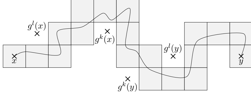
FIGURE 3.4. Construction de l'ensemble D
