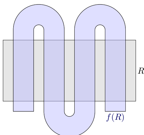
FIGURE 3.3. 4-fer à cheval de Smale
