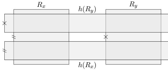
FIGURE 3.5. Construction de l'homéomorphisme h
