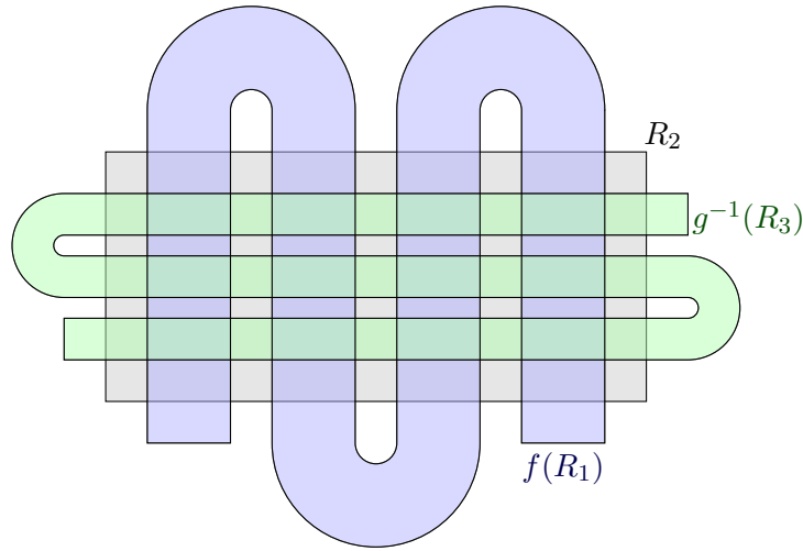
FIGURE 3.2. Intersection de f(R_1) et g^{-1}(R_3)
