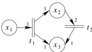
FIG. 1 – Un réseau de Petri.
