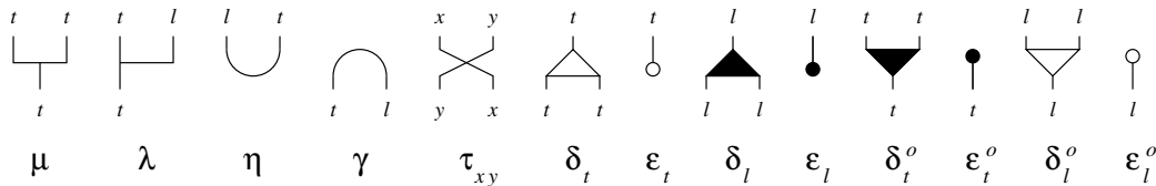
FIG. 6.6 – Une signature à 16 générateurs.
