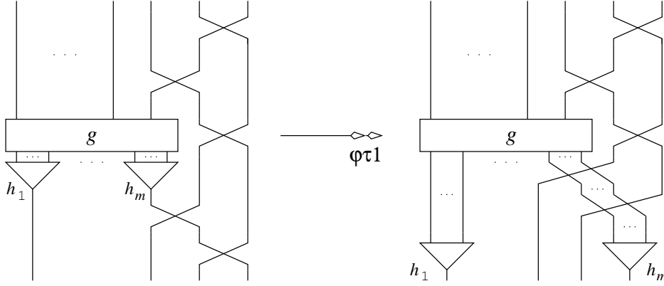
FIG. 5.10 – Réduction d'une paire critique indexée par une R_{\Delta, \Sigma} -forme normale f = (h_1 \otimes \dots \otimes h_m) \circ g de \mathcal{L}\Sigma^c à une paire critique indexée par une R_{\Delta} -forme normale g de \mathcal{L}\Delta .
