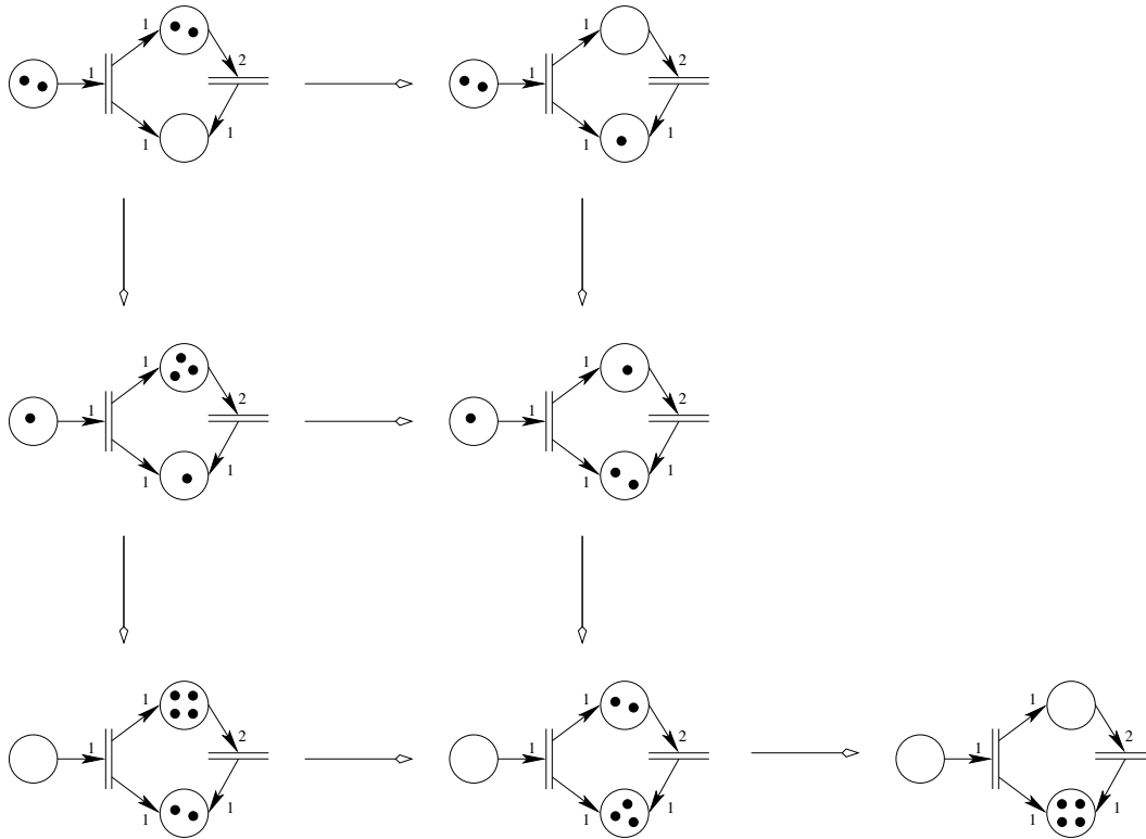
FIG. 2 – Les évolutions possibles d'un état du réseau.
