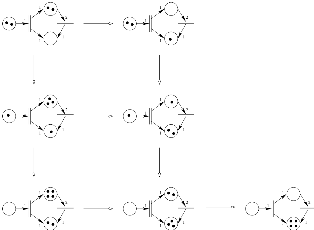
FIG. 4.2 – Évolutions possibles d'un marquage d'un réseau de Petri.
