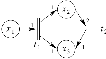
FIG. 4.1 – Un exemple de représentation graphique associée à un réseau de Petri.
