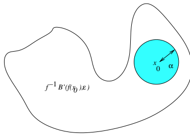
FIG. 2 – L'image inverse de B'(f(x_0), \epsilon) contient une boule B(x_0, \alpha)
